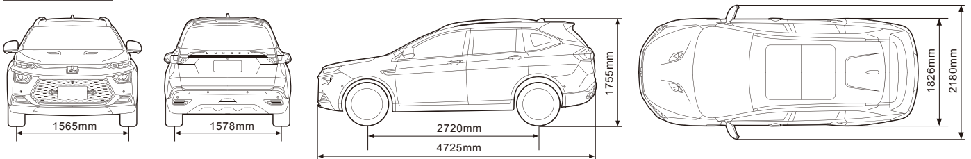
規格圖
